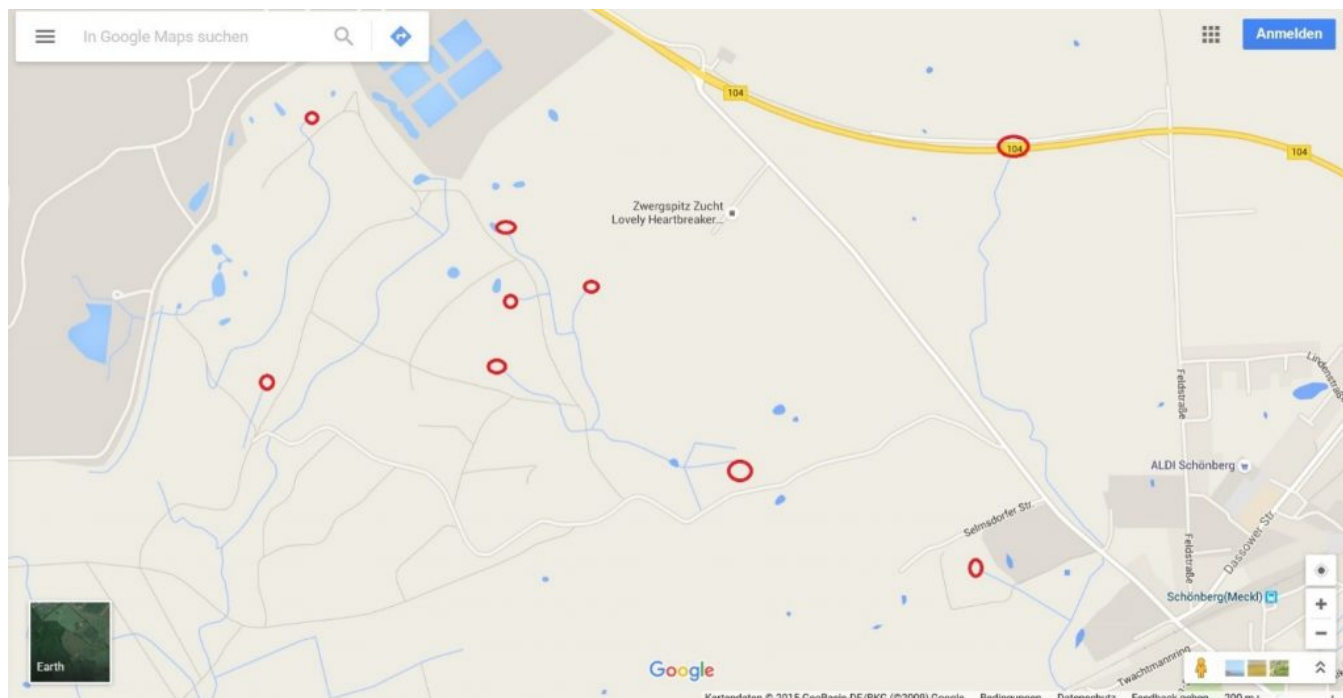
Wasseraustritte Südhang des Ihlenberg Richtung Schönborg © Google Maps
