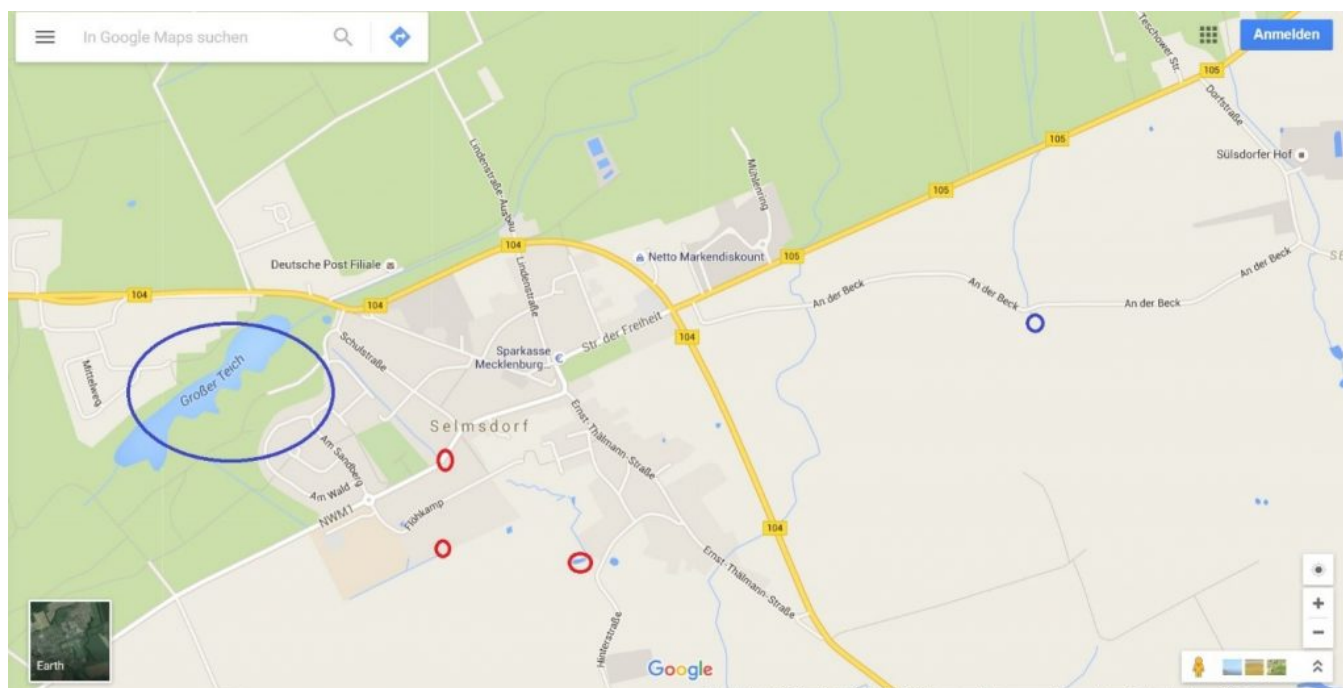
Wasseraustritte Nordhang des Ihlenberg Richtung Selmsdorf © Google Maps
